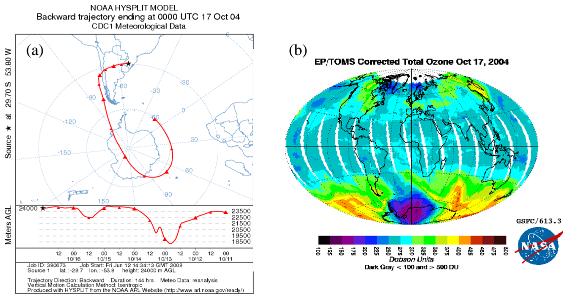
Fig. 6.8 - (a) Origem da trajetória das massas de ar para o dia 17 e para os 6 dias anteriores de 17 de outubro de 2004 e em (b) imagem de satélite mostrando o deslocamento, no dia 17 de outubro de 2004, de massa de ar do Buraco de Ozônio Antártico para o Sul do Brasil.
