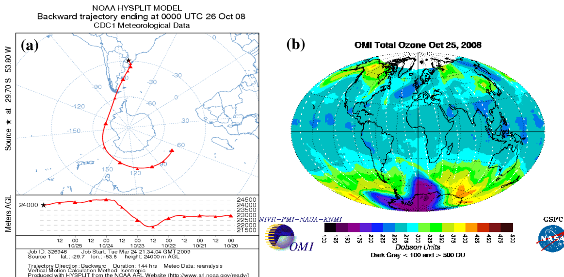
Fig. 6.14 - (a) Origem da trajetória das massas de ar para o dia 26 e para os 6 dias anteriores de 26 de outubro de 2008 e em (b) imagem de satélite mostrando a passagem, no dia 25 de outubro de 2008, de massa de ar do Buraco de Ozônio Antártico sobre o Sul do Brasil.
