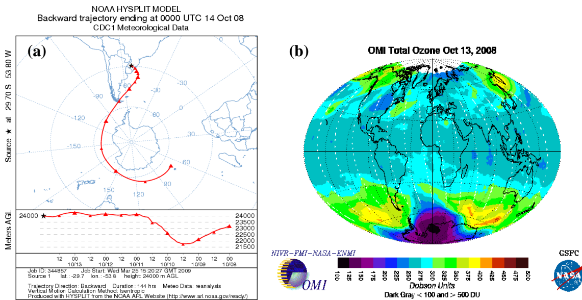
Fig. 6.12 - (a) Origem da trajetória das massas de ar para o dia 14 e para os 6 dias anteriores de 14 de outubro de 2008 e em (b) imagem de satélite mostrando o deslocamento de massa de ar do Buraco de Ozônio Antártico para o Sul do Brasil, no dia que antecede a queda de ozônio, dia 13 de outubro 2008.
