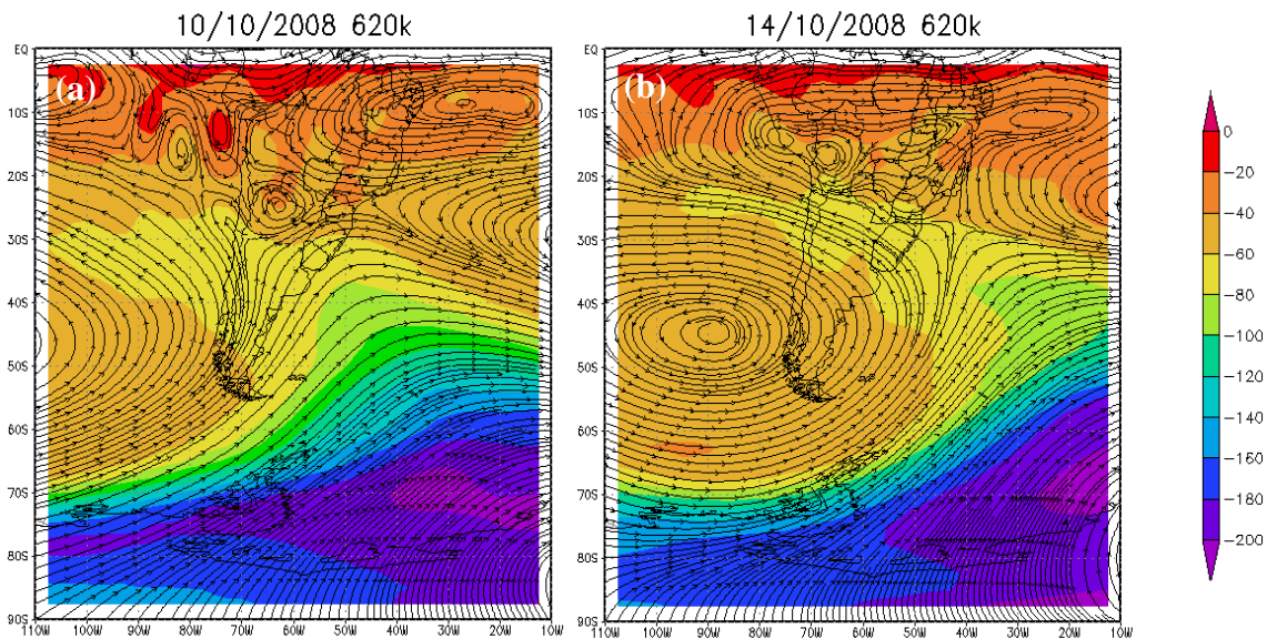
Fig. 6.11 - Vorticidade potencial com campos de vento sobrepostos em superfícies isentrópicas indicando o possível movimento das massas de ar em (a) no dia 10 de outubro de 2008 e em (b) no dia 14 de outubro de 2008 a 620K.
