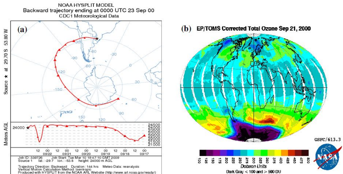
Fig. 6.4 - (a) Origem da trajetória das massas de ar para o dia 23 e para os 6 dias anteriores de 23 de setembro de 2000 e em (b) imagem de satélite mostrando para o dia 21 de setembro de 2000 a aproximação de massas de ar do Buraco de Ozônio Antártico para o Sul do Brasil.
