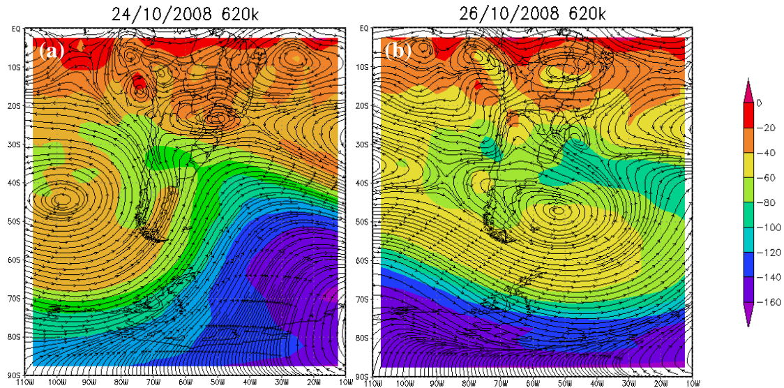
Fig. 6.13 - Vorticidade potencial com campos de vento sobrepostos em superfícies isentrópicas indicando o possível movimento das massas de ar em (a) no dia 24 de outubro de 2008 e em (b) no dia 26 de outubro de 2008 a 620K.
