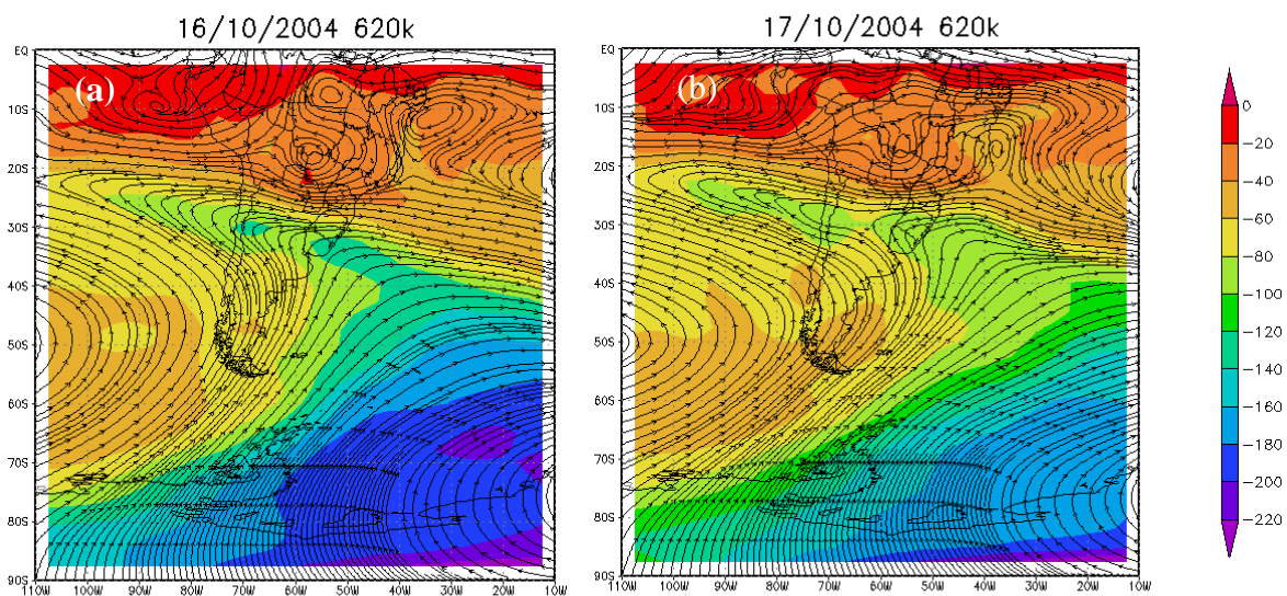
Fig. 6.7 - Vorticidade potencial com campos de vento sobrepostos em superfícies isentrópicas indicando o possível movimento das massas de ar em (a) no dia 16 de outubro de 2004 e em (b) no dia 17 de outubro de 2004 a 620K.
